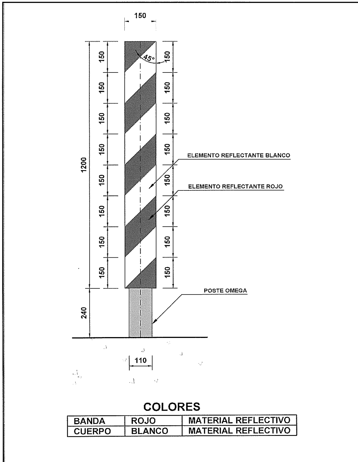
FIGURA 6.305.7.A DELINEADOR VERTICAL DERECHO
