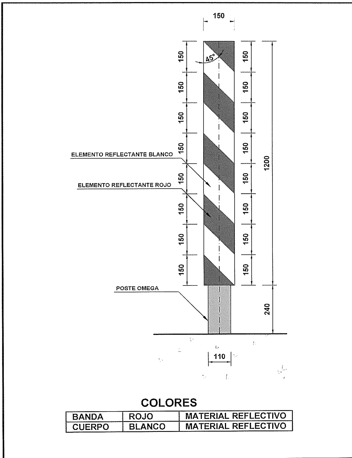
FIGURA 6.305.7.B DELINEADOR VERTICAL IZQUIERDO
